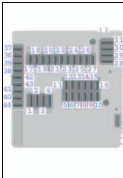
Caja de fusibles, parte delantera
